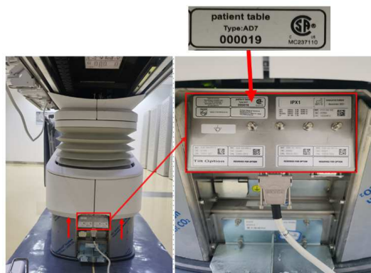
Slika 2. Mesto oznak na mizi z mizo v najvišjem položaju (leva stran) in oznaka z vrsto mize (desna stran)
